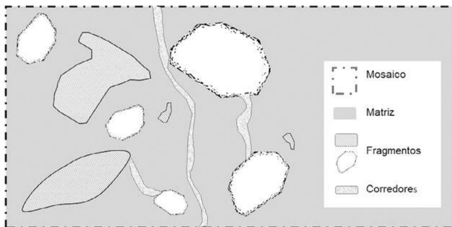
Figura 4.1. Esquema del modelo de paisaje “Mosaico: Matriz – Parche – Corredor”. Fuente: Armenteras & Vargas 2016
