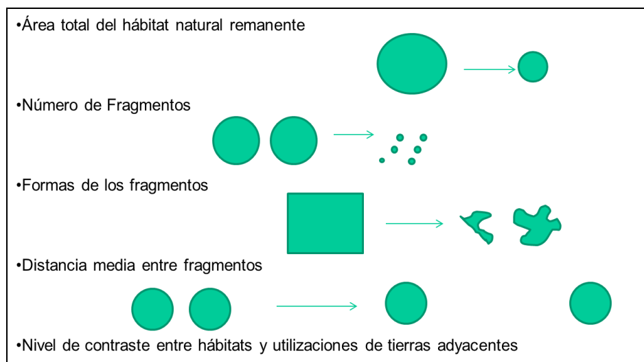
Figura 4.2. Principales patrones del paisaje para medir fragmentación
