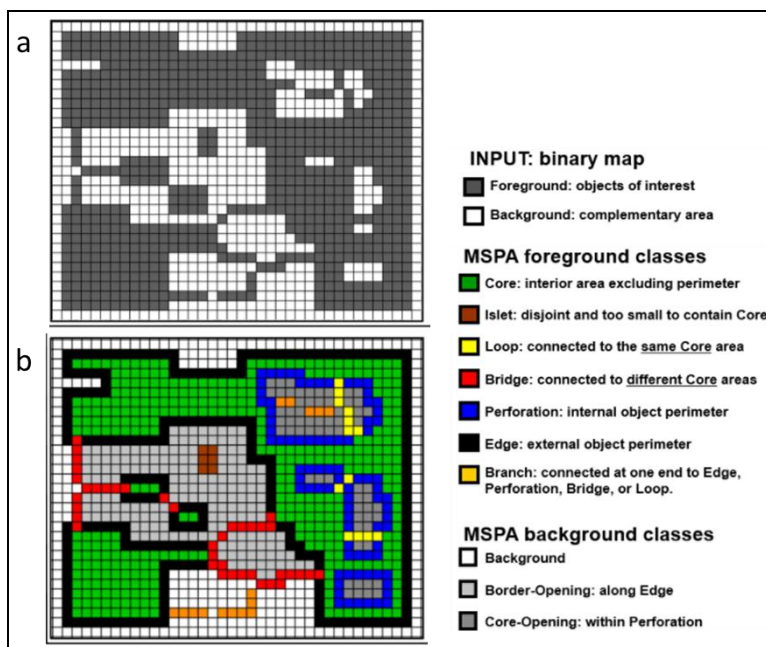
Figura 6.2. Imágenes de entrada (a) y salida (b) para el análisis MSPA. Fuente: sitio web MSPA 19
